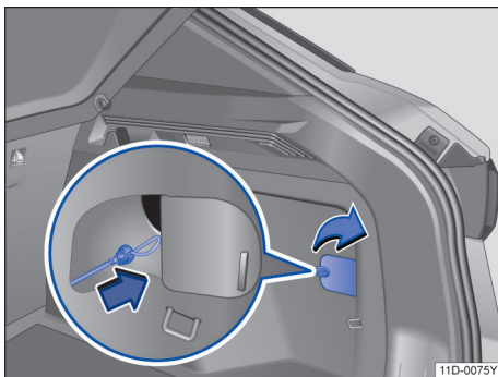
图 139 行李厢内的交流充电插头应急解锁拉索
