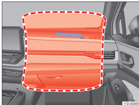
图 29 副驾驶前部安全气囊的安装位置和膨胀范围
