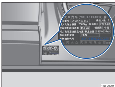
图 165 B 柱下方整车产品标牌
