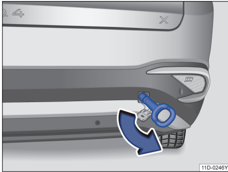
图 153 在保险杠右后部：安装牵引环
