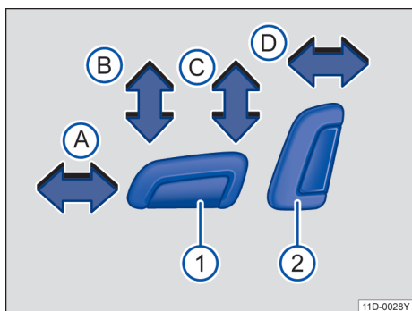
图 61 调整座椅的前后位置、座椅面的高度和倾斜角度
