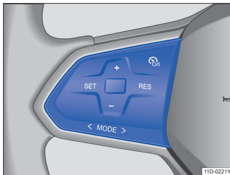
图 96 多功能方向盘左侧：定速巡航系统操作按钮
