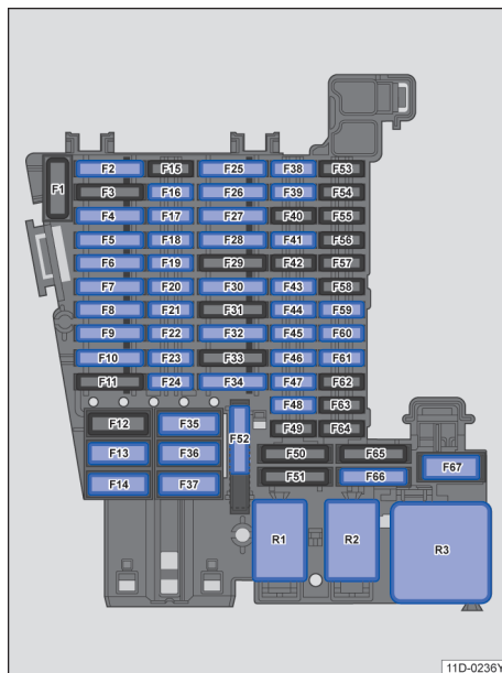
图 145 保险丝位置示意图
