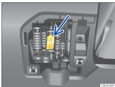
图 146 救援用保险丝
