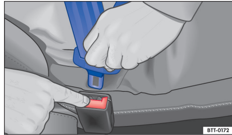
图 24 从插口上松开安全带锁舌
