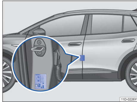
图 162 车辆 B 柱上：胎压标签
