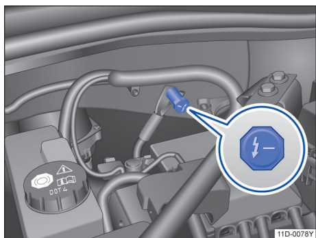
图 148 车身上的负极（接地点）
